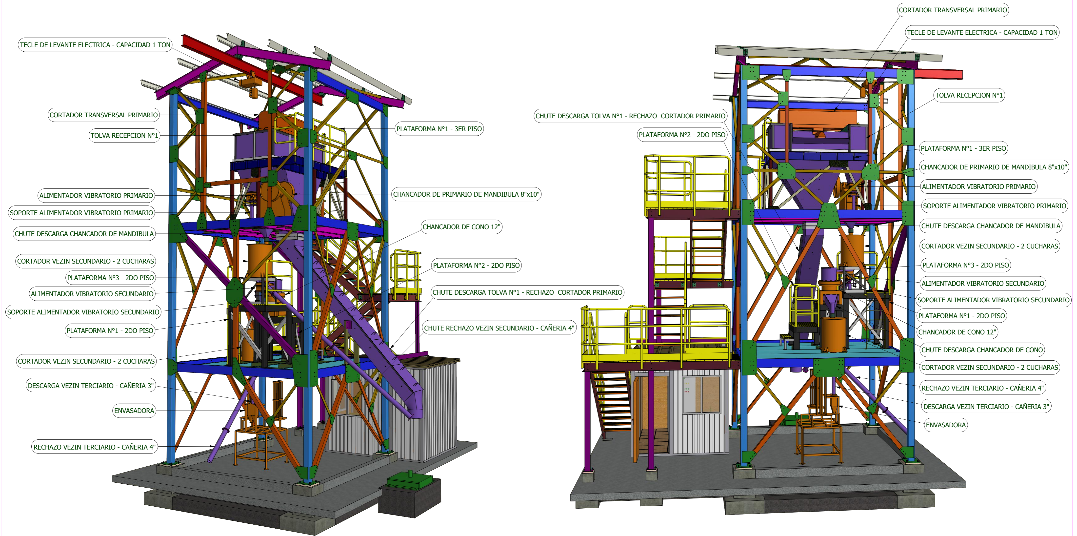
VISTA PERSPECTIVA DIPOSICION DE EQUIPOS INTERIOR TORRE MUESTRERA 1A ESC: 1:50
